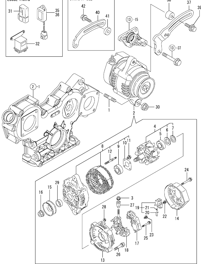
Fig.19. GENERATOR
